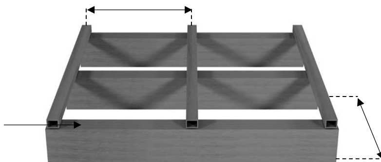
Rysunek 3. Legary aluminiowe na konstrukcji stalowej
