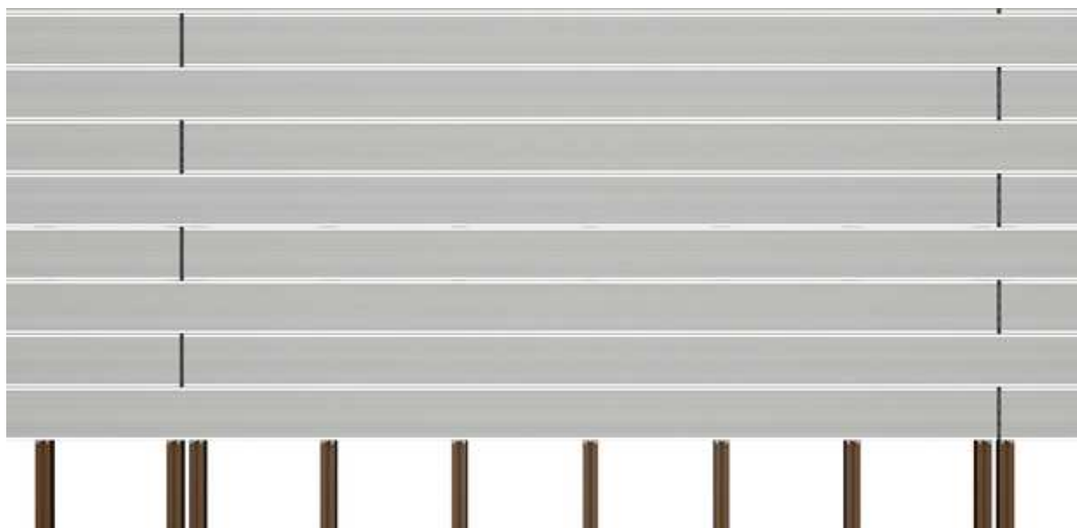
Rysunek 11. Układ legarów przy czołowym połączeniu desek - taras na tzw. mijanę
