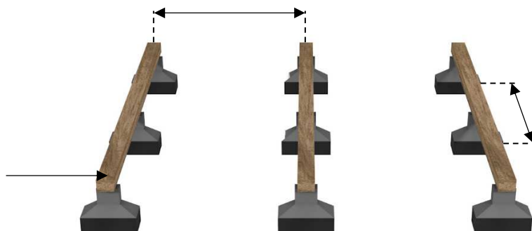
Rysunek 4. Legary drewniane na wspornikach poziomujących z tworzyw sztucznych
