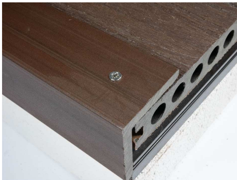
Rysunek 21. Montaż listwy za pomocą wkrętów samowiercących od strony bocznej desek
