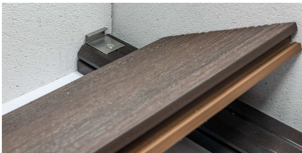
Rysunek 14. Montaż pierwszej deski na klipsie startowym
