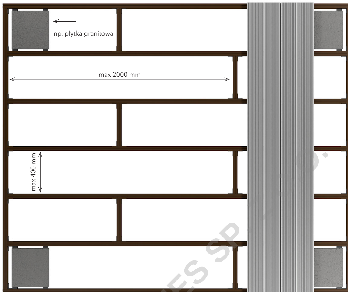
Rys 7. Taras pływający - rama z legarów połączona kątowymi łącznikami ciesielskimi, obciążona płytami betonowymi
