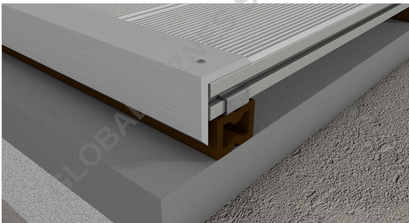
Rys 23. Montaż listwy za pomocą wkrętów samowiercących od strony czołowej desek
