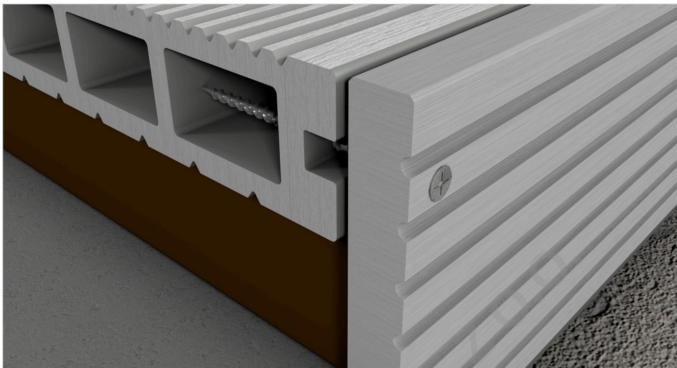
Rys 18. Montaż listwy za pomocą wkrętów samowiercących
