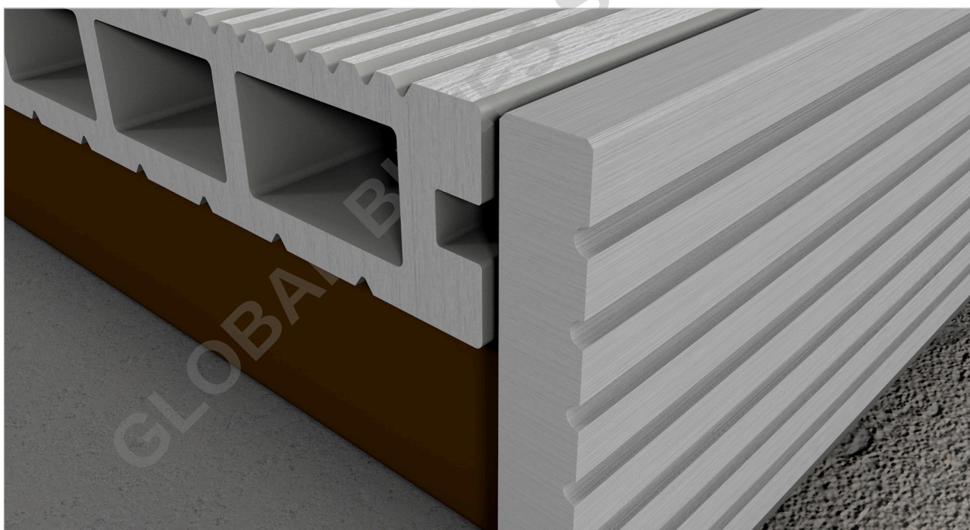
Rys 19. Montaż listwy za pomocą kleju elastomerowego
