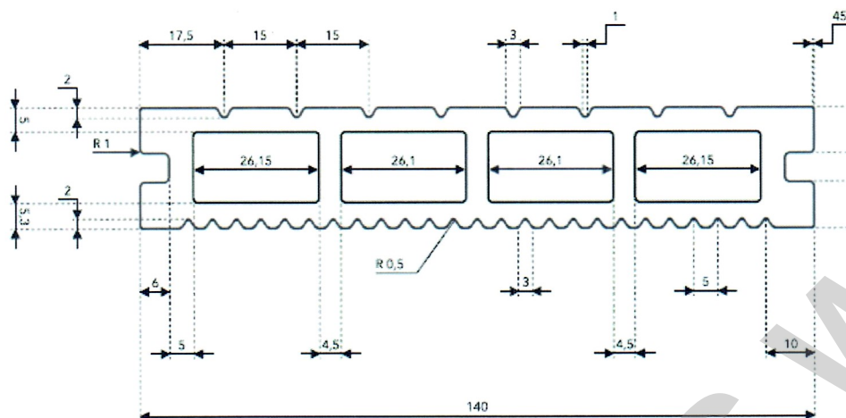
Rysunek A1. Deska tarasowa
