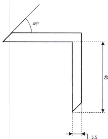
Rysunek A4. Listwa kątowna
