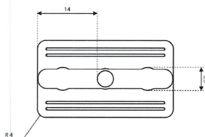
Rysunek A6. Klips montażowy tworzywowy
